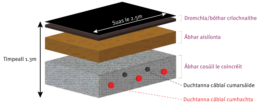
Fíor 10: Gnáthshocrú duchta le haghaidh cábla HVAC faoin talamh
